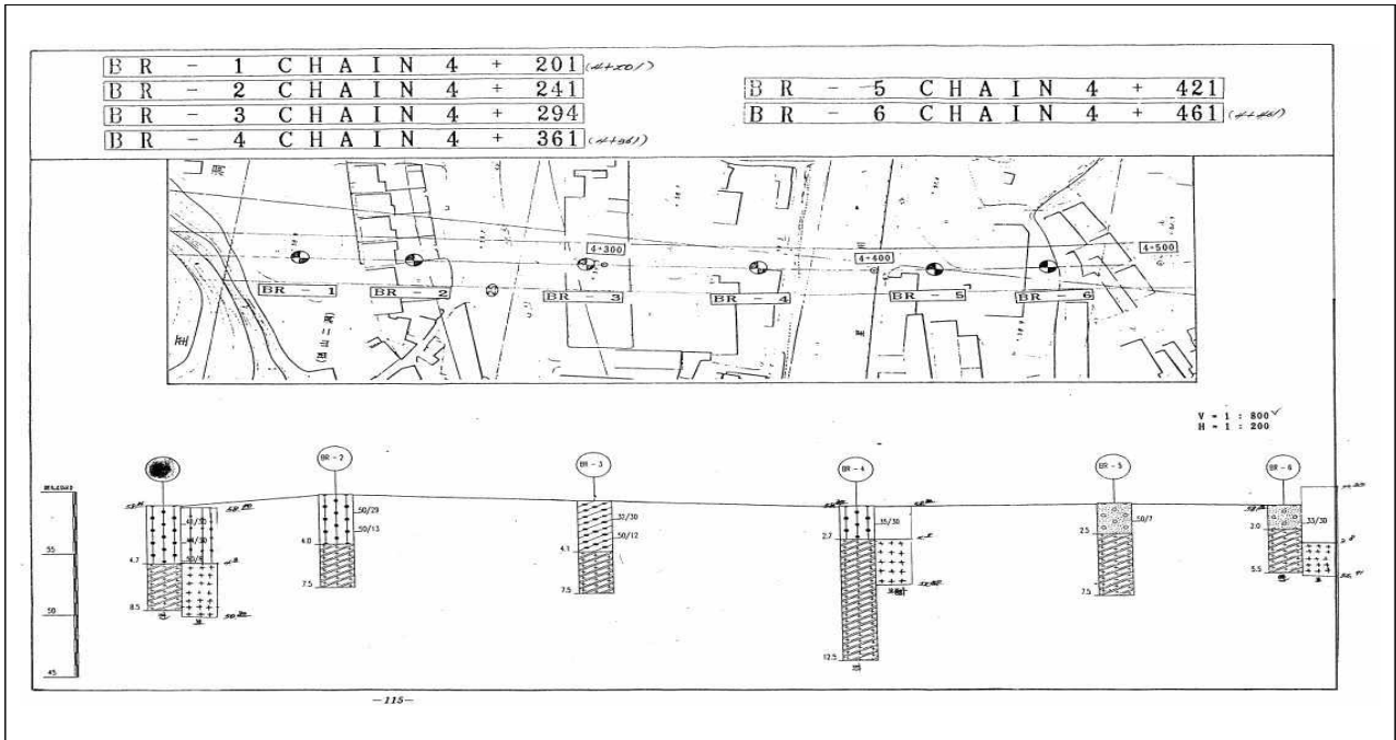
【그림 2.2.1】 시지교 토질조사 위치
